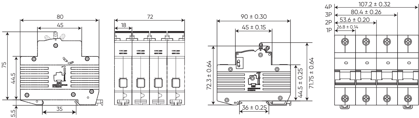
SERI MP4 - MP6: 6A - 63A
